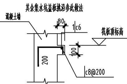
集水坑侧边遇混凝土墙时挑沿构造
