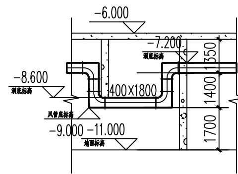
下翻风管剖面示意图
