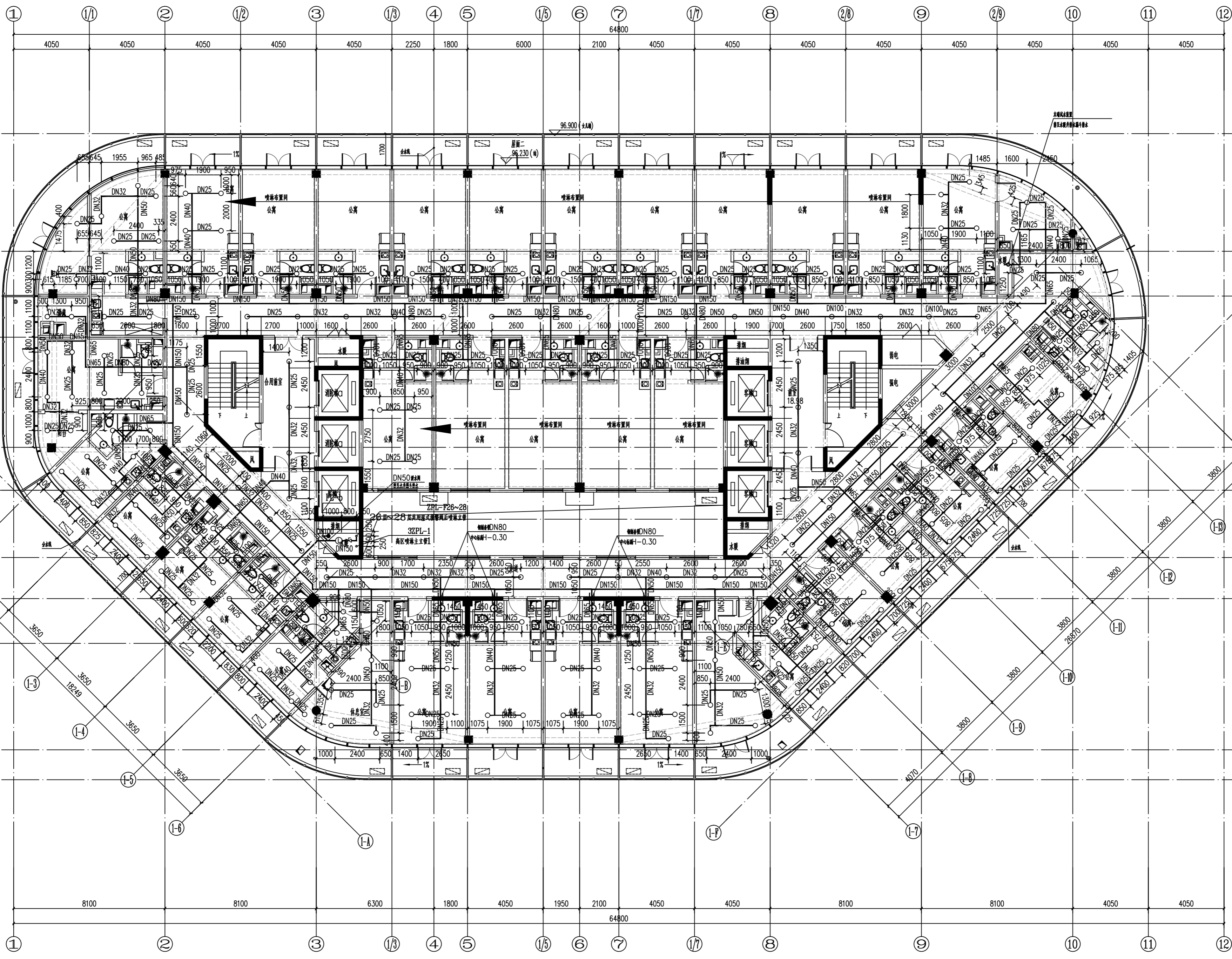
二十八层自动喷淋平面图 1:100 本图面积411.68m 2 ，共38#
