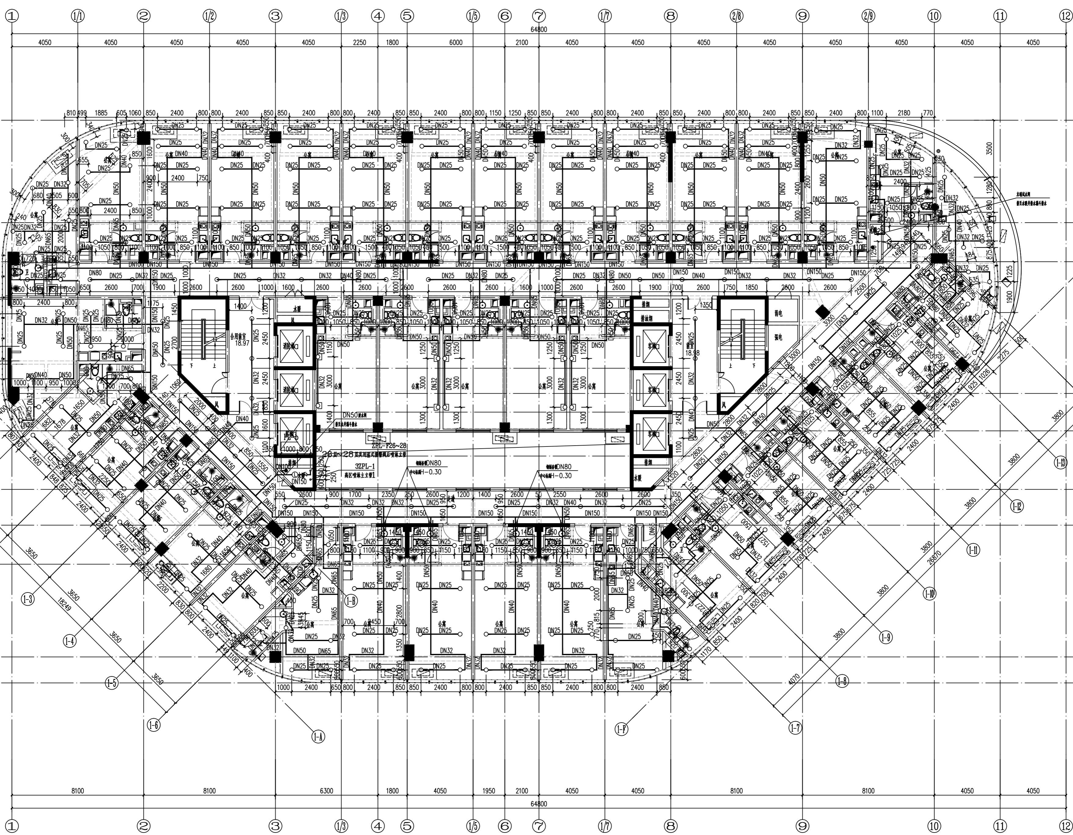
二十七层自动喷淋平面图 1:100 本图面积676.03m 2 ，共38#
