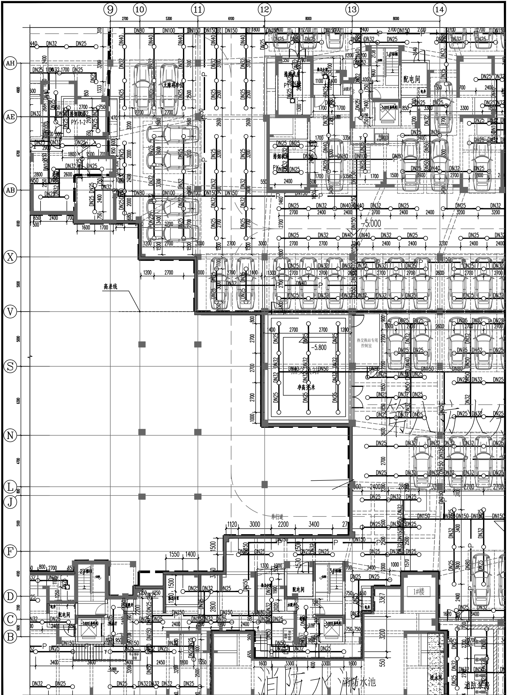
附图2: 项目名称 山水文苑 工程名称 地下车库 设计编号 HNGH-XM-2019-2706-16 变更号 03 第3页
