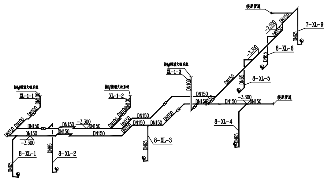
消火栓系统图修改
