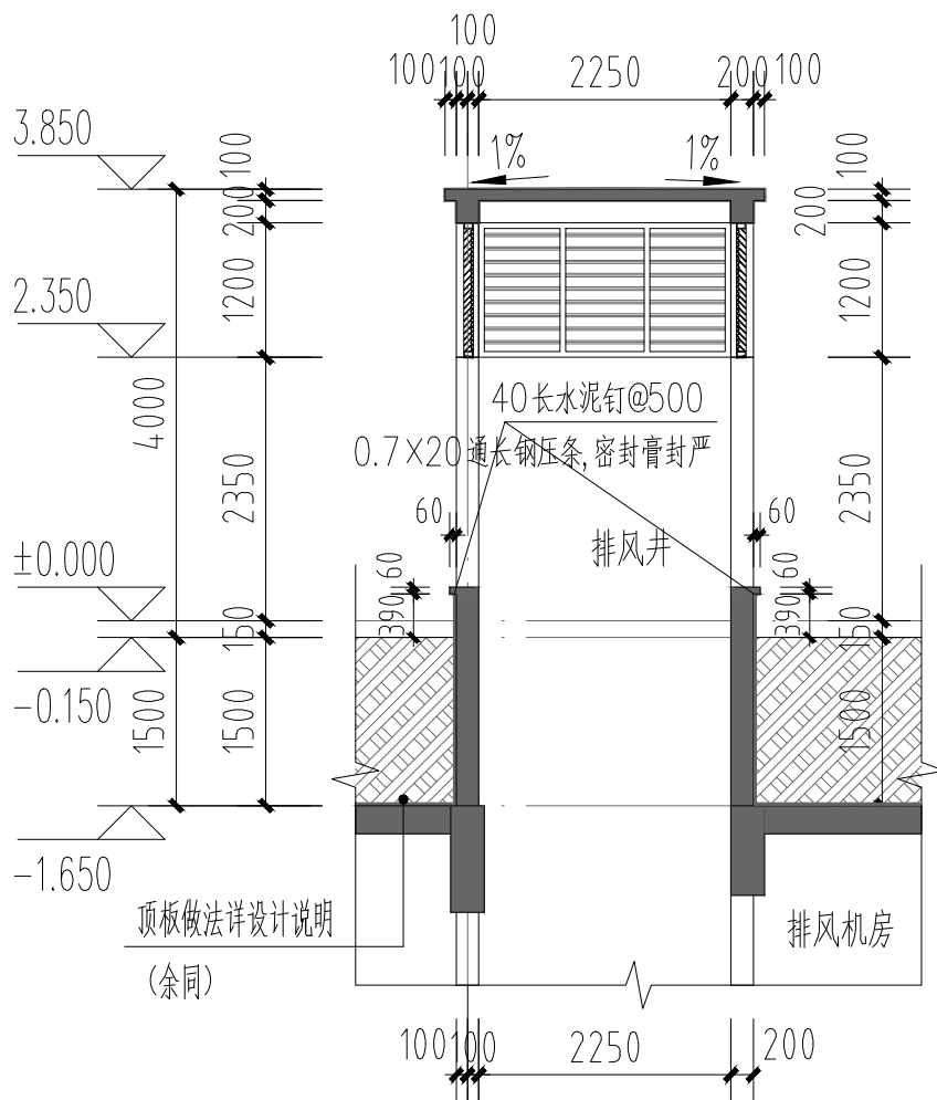
1-K a-a 剖面图
