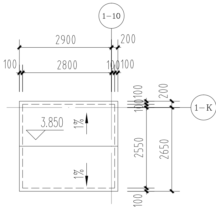
地下车库排风井屋顶平面图 1:100
