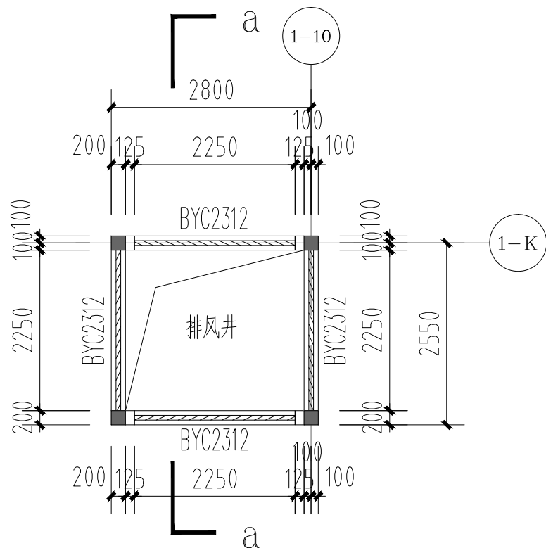
地下车库排风井平面图 1:100
