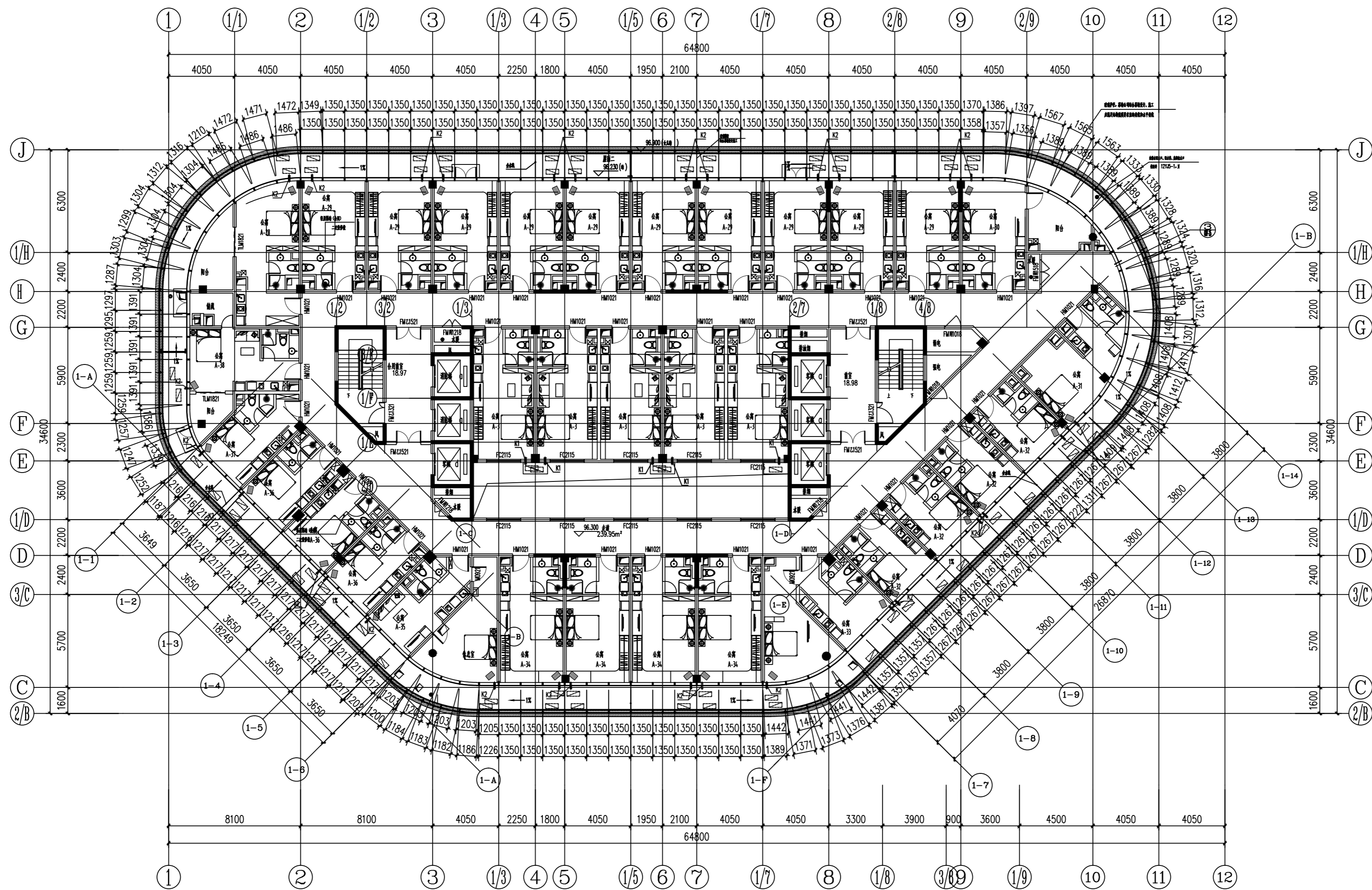
二十八层平面图
