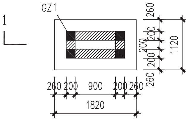
图1 装饰柱基础平面图
