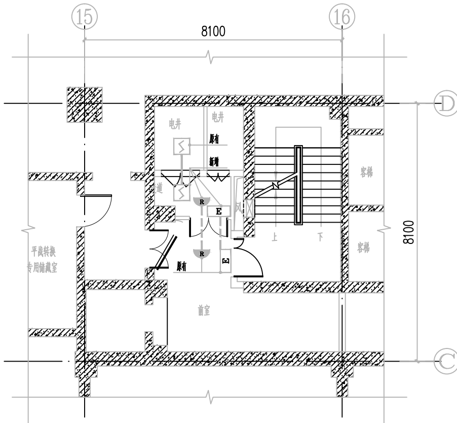
地下一层、地下二层局部电气平面图 1:100
