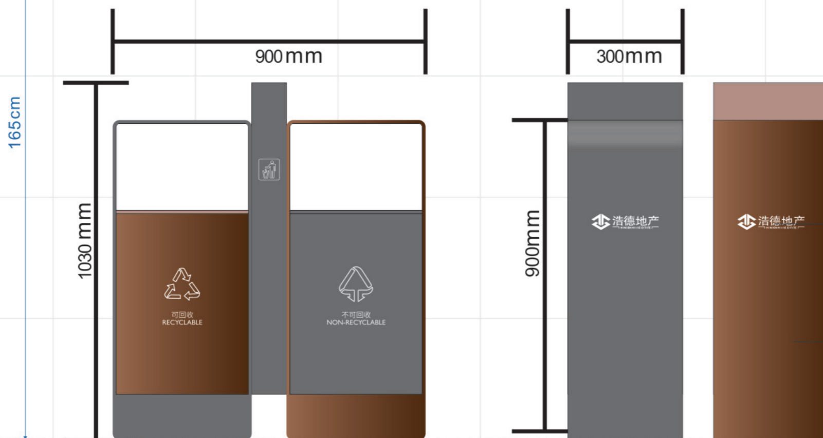
正视图
