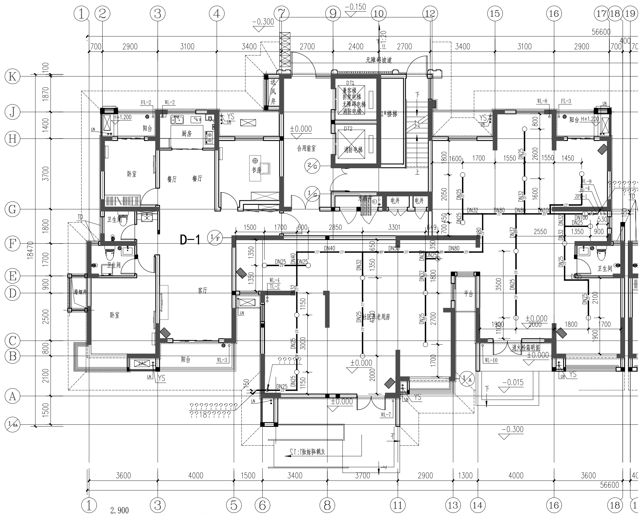
附图1: 养老服务用房自喷修改平面图 1:100
