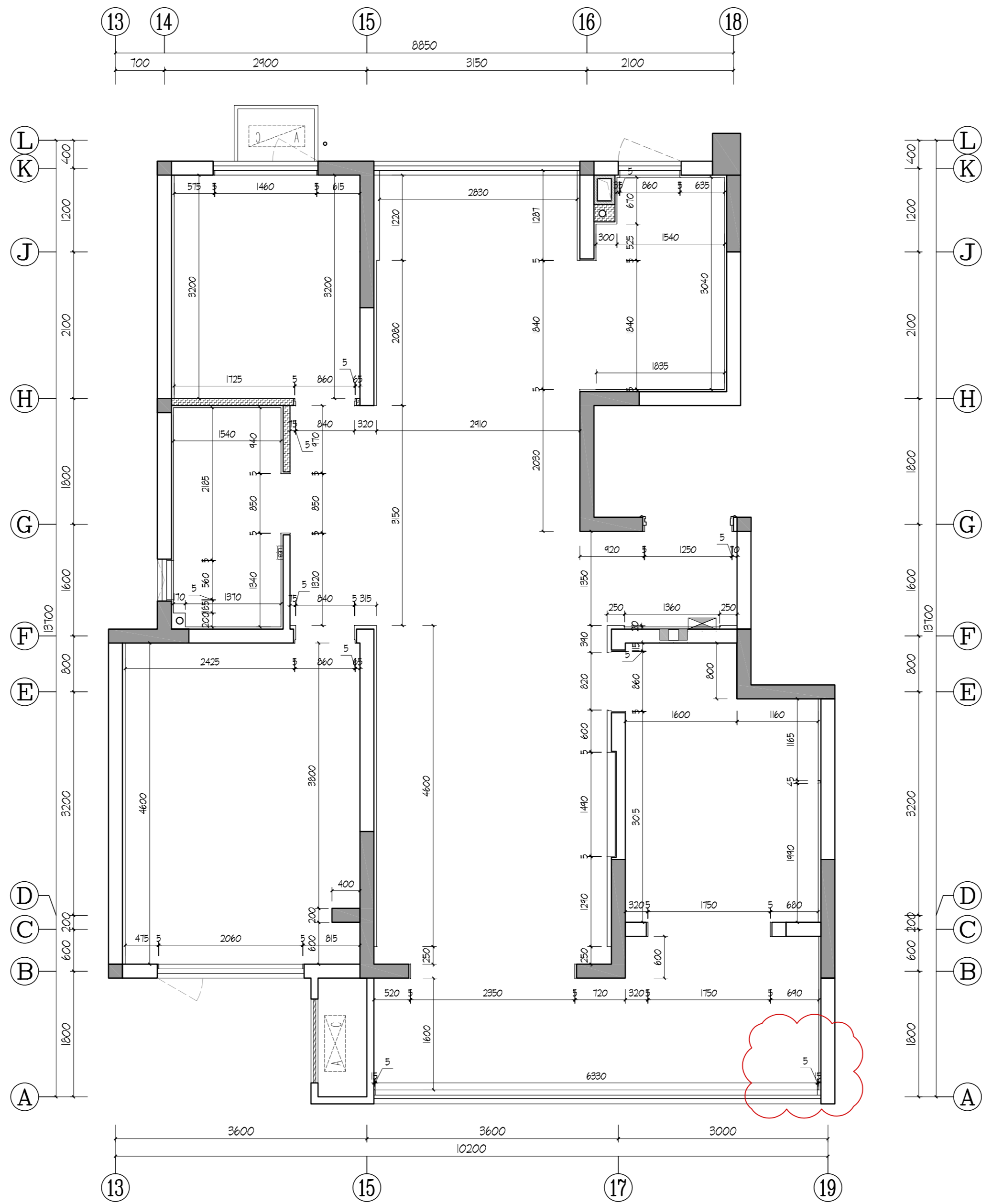
01 SURFACE DIMENSION PLAN 完成面尺寸图 SCALE 1: 50
