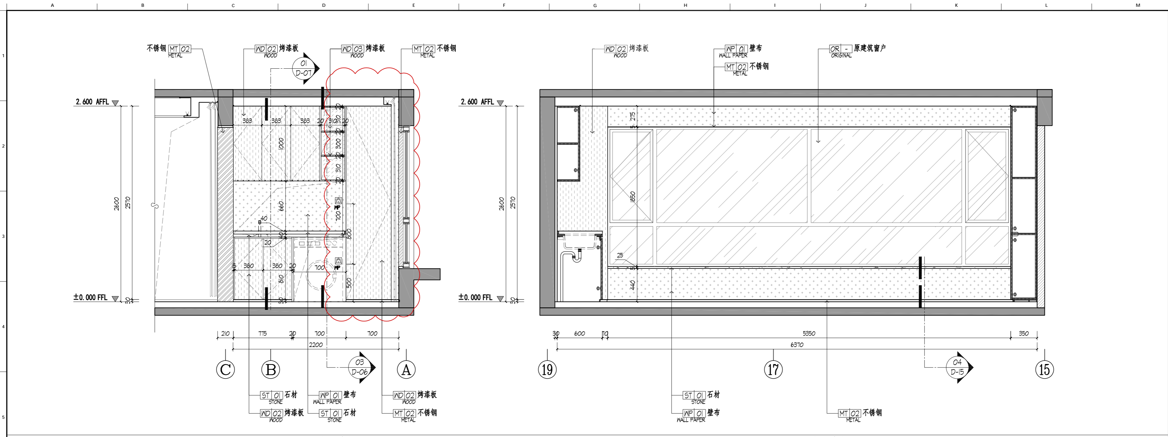
11 ELEVATION 立面图 P-16 SCALE 1: 30
