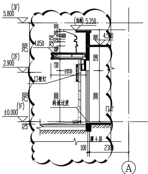
剖面图 1:100
