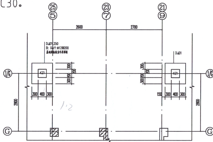
门厅一层平面图 1:50
