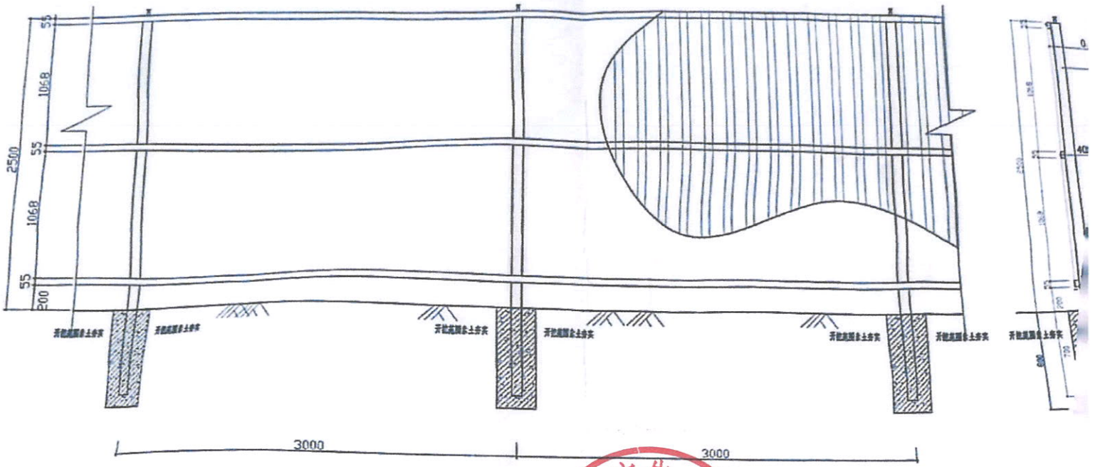
2.5m 围墙立面图
