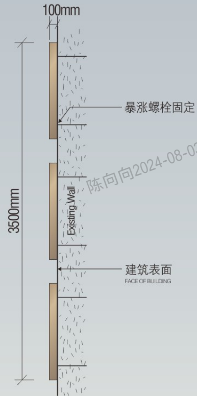
2 侧立面 - Side Elevation 1:10
