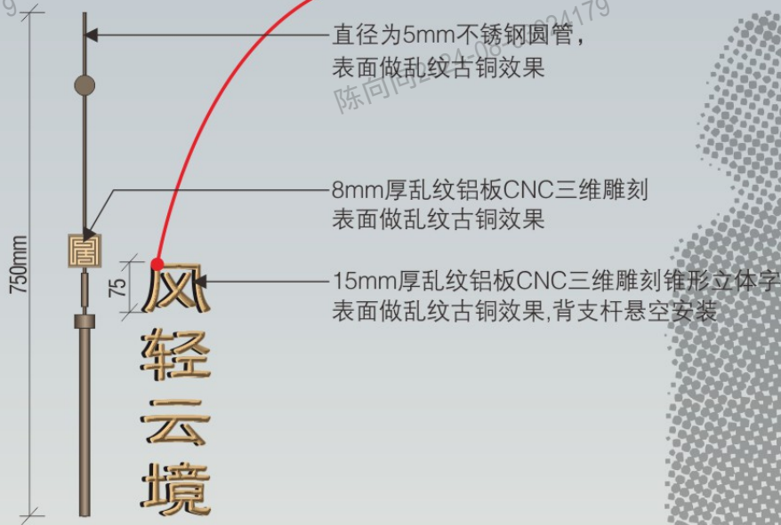
1 正立面-Front Elevation 1:10
