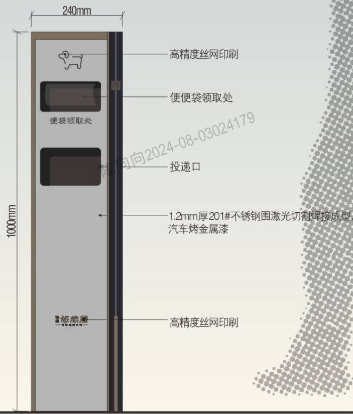
1 正立面-Front Elevation 1:10
