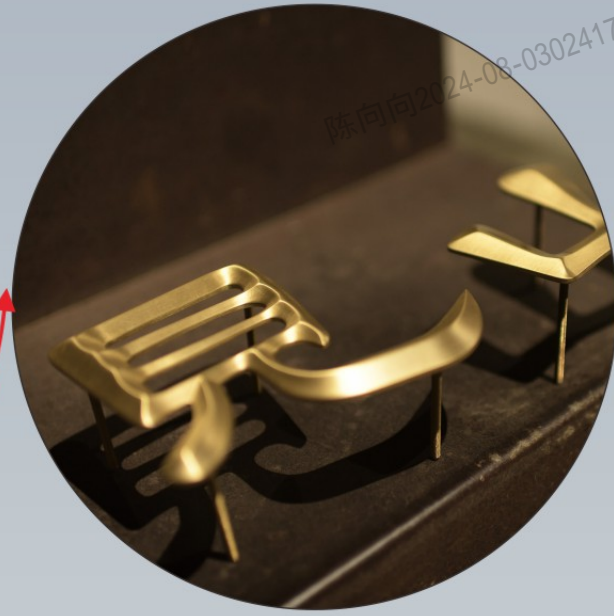
15mm厚乱纹铝板CNC三维雕刻锥形立体字 表面做乱纹古铜效果
