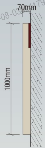
2 侧立面 - Side Elevation 1:10
