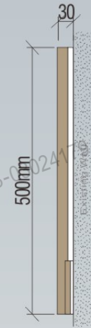
2 侧立面 - Side Elevation 1:10
