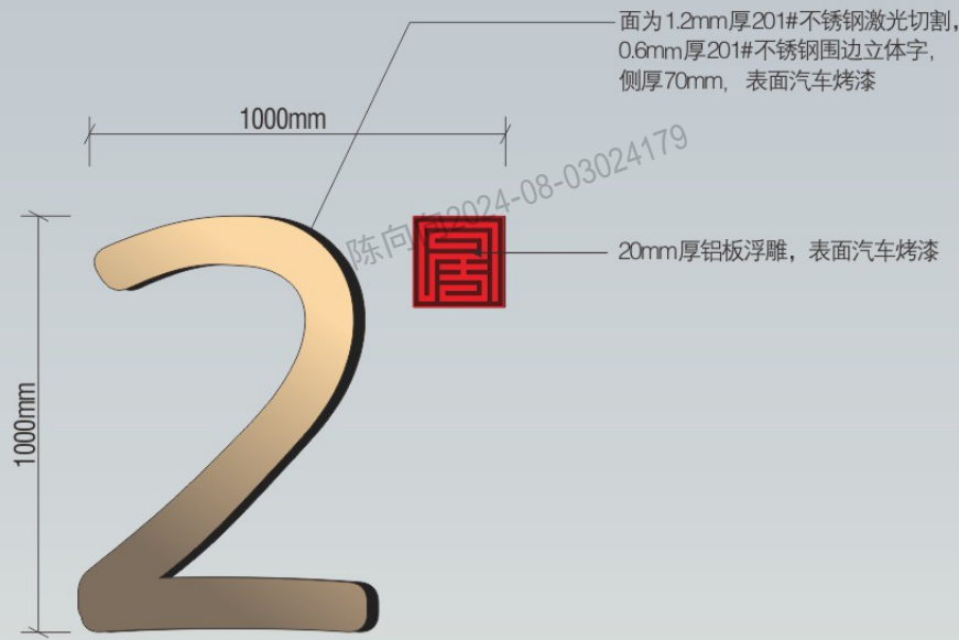
1 立面 - Elevation 1:10
