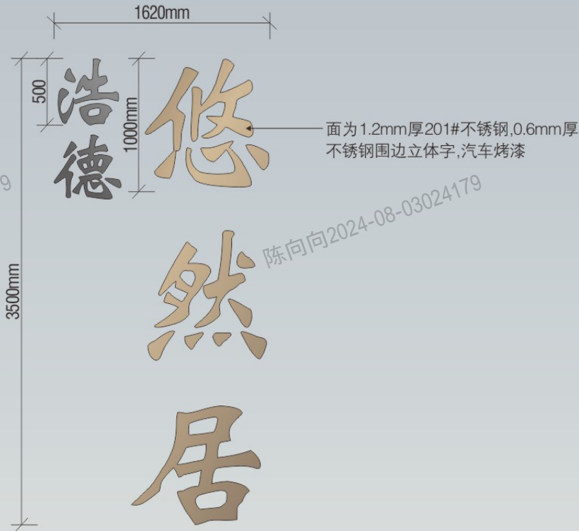
1 正立面 - Front Elevation 1:10
