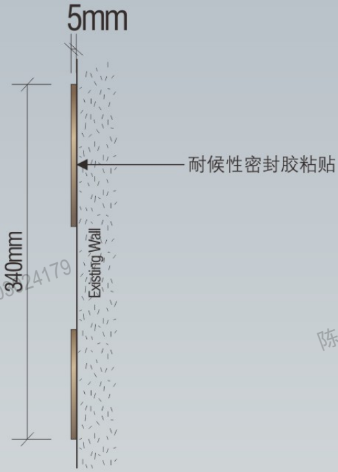
2 侧立面 - Side Elevation 1:5
