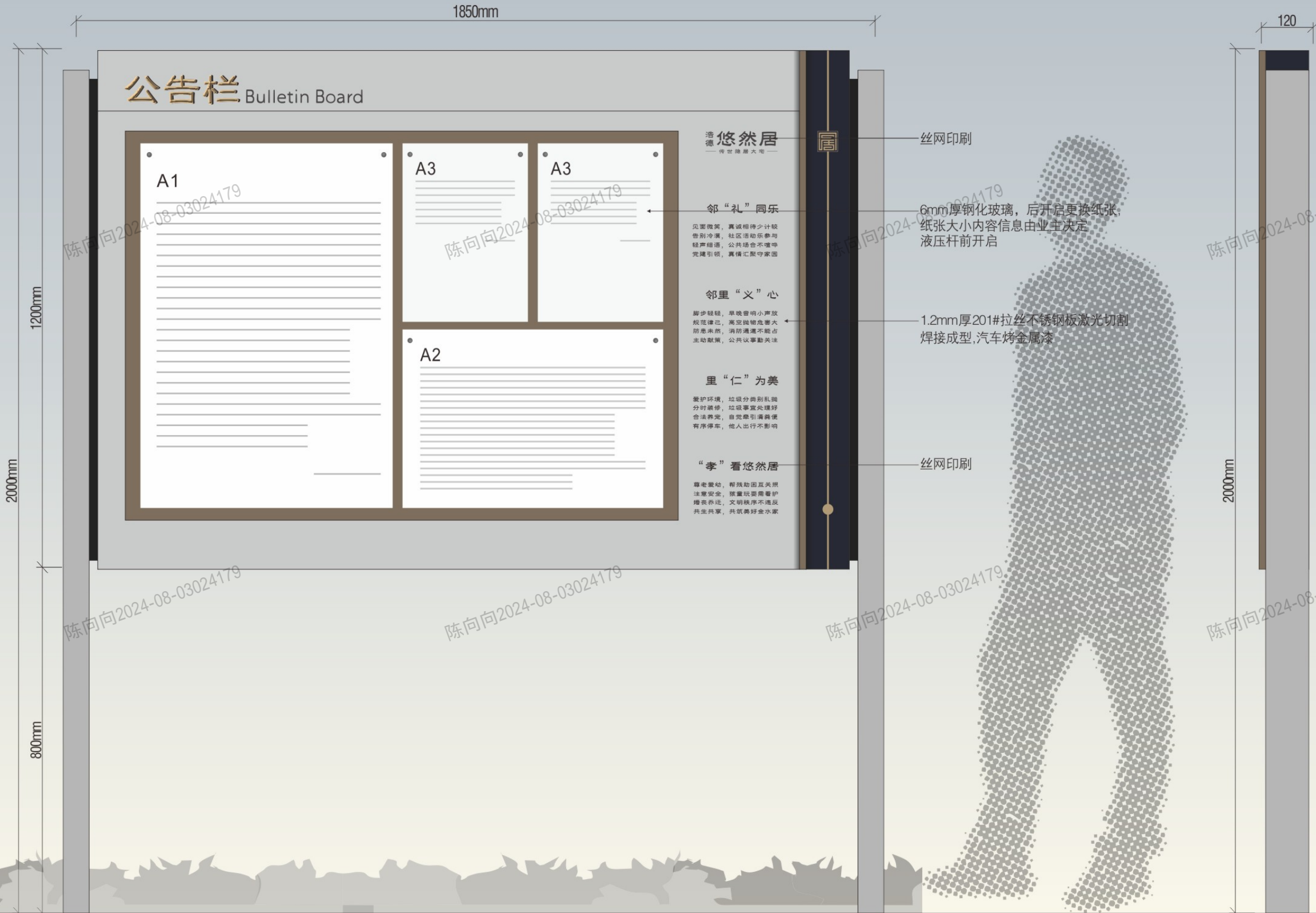
1 正立面-Front Elevation 1:10
