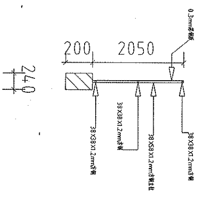
3-3 剖面图
