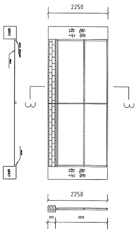
地下室围墙立面图
